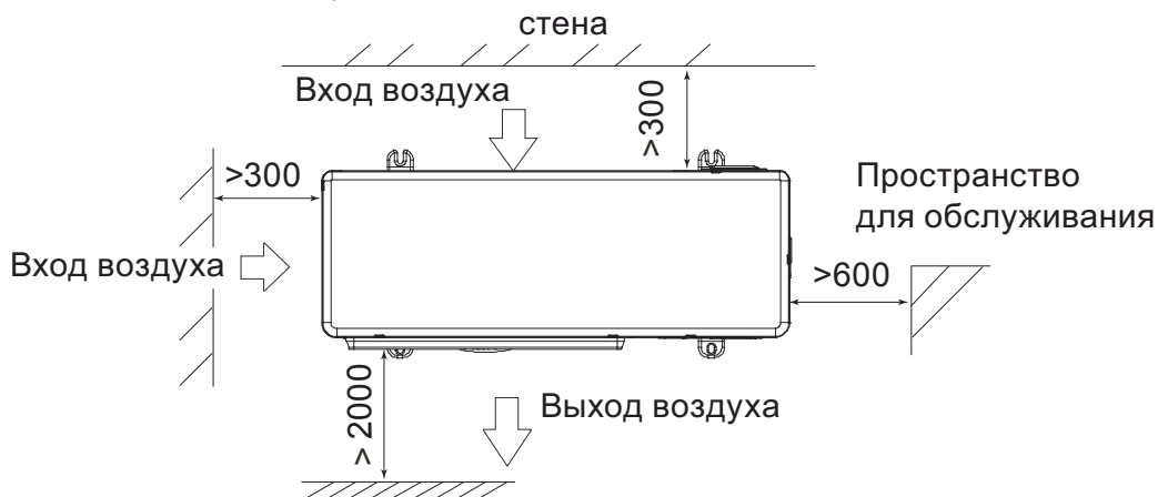
Одиночный наружный блок
