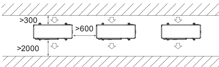
Монтаж нескольких наружных блоков в ограниченном пространстве
