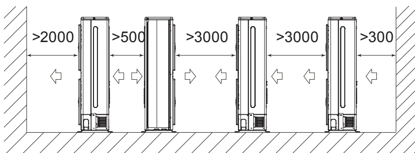
Монтаж нескольких наружных блоков в ограниченном пространстве
